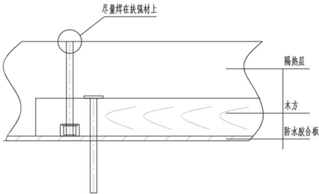
图2 防冷桥吊点示意图
